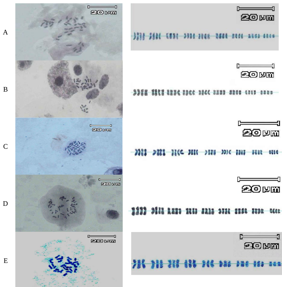
شکل ۱- کاریوتیپ و پهنه میتوزی جمعیت‌های مختلف گونه C. dactylon . A: جمعیت ۱، B: جمعیت ۶، C: جمعیت ۱۶، D: جمعیت ۲۹، E: جمعیت ۳۳.
