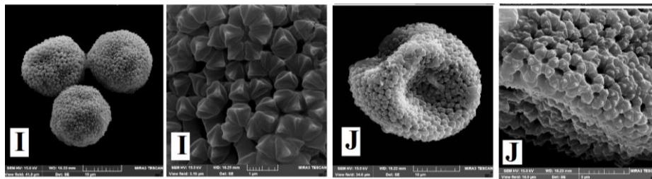
شکل ۲- تصاویر دانه‌گرد جمعیت‌های مطالعه‌شده با میکروسکوپ الکترونی SEM؛ A. D. mucronata (کرمانشاه)، B. D. mucronata (کردستان)، C. D. mucronata (اراک)، D. D. mucronata (همدان)، E. D. mucronata (لرستان)، F. D. mucronata (لرستان)، G. D. oleoids (کردستان)، H. D. oleoids (کرمانشاه، بیستون)، I. D. oleoids (کرمانشاه، محمودآباد)، J. D. pontica (ساری، سنگده) از نمای قطبی - نمای استوایی.
